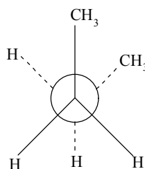
Gauche form
