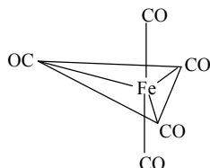
Pentacarbonyl iron (0) \text{Fe(CO)}_5
